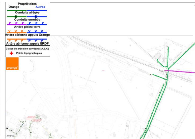
Figure 76 : Plan des réseaux de télécommunication ORANGE aériens et souterrains (Source : ORANGE)
