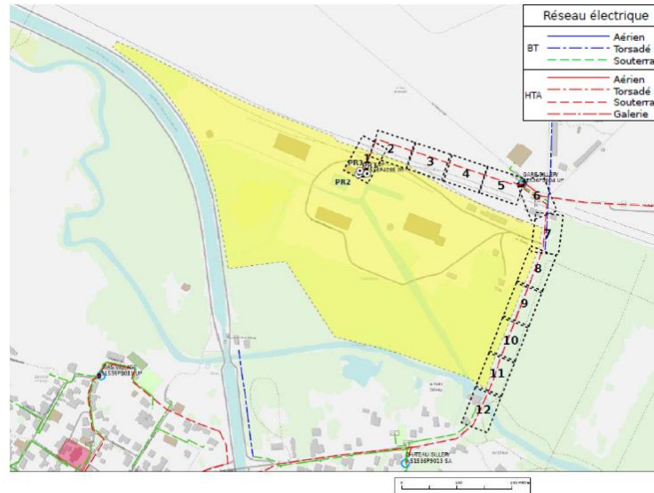
Figure 75 : Plan d'ensemble des réseaux électriques aériens et souterrains (Source : ENEDIS)
